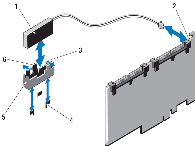
图 3-15. 卸下和安装 RAID 电池
