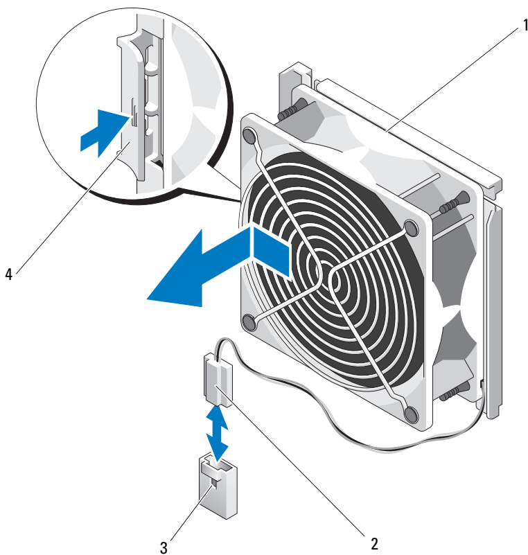
图 3-21. 卸下和安装系统风扇
