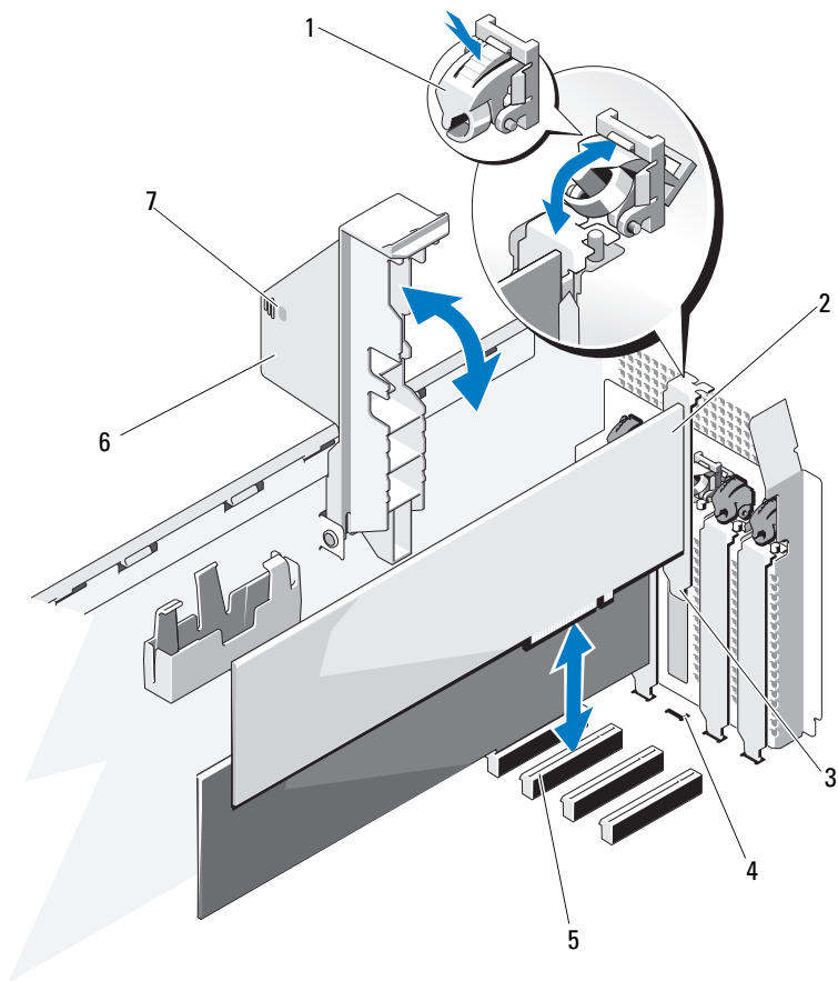
图 3-14. 卸下和安装扩充卡
