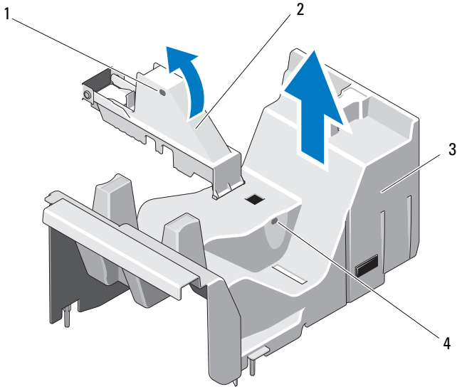
图 3-6. 卸下和安装冷却通风罩
