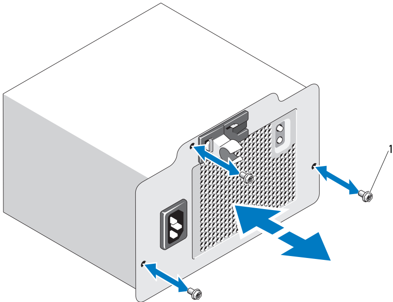
图 3-17. 卸下和安装非冗余电源设备
