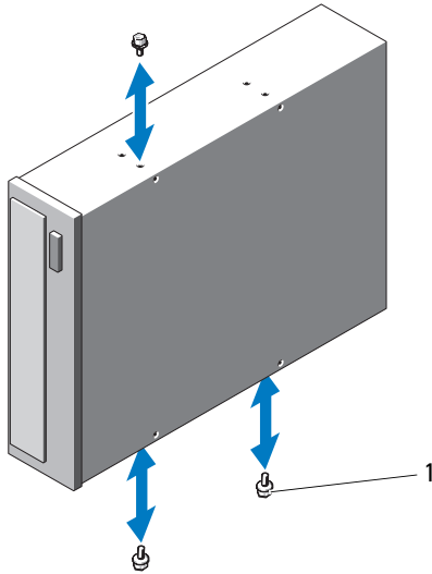
图 3-12. 安装光盘驱动器或磁带驱动器轴肩螺钉
