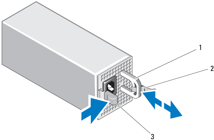
图 3-16. 卸下和安装冗余电源设备
