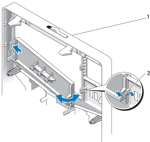
图 3-3. 卸下和安装前挡板插件
