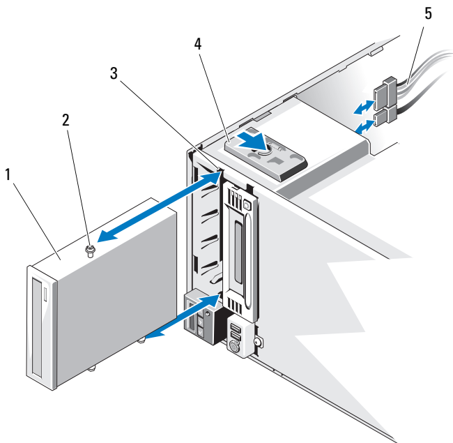
图 3-11. 卸下和安装光盘驱动器或磁带驱动器
