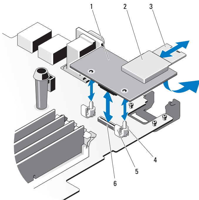
图 3-20. 卸下和安装 iDRAC6 Enterprise 卡
