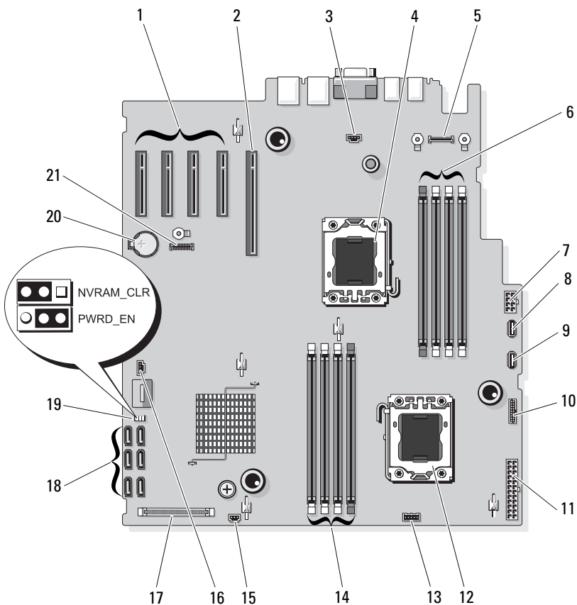
图 6-1. 系统板跳线和连接器
