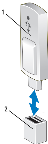
图 3-18. 卸下或安装 USB 存储钥匙
