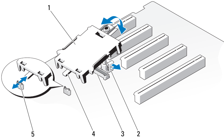
图 3-19. 卸下和安装 iDRAC6 Express 卡
