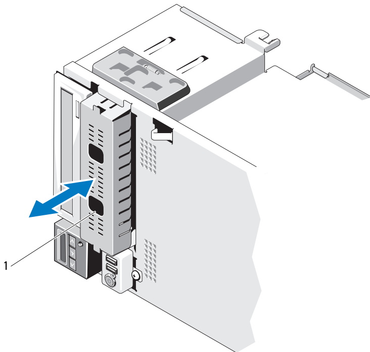
图 3-4. 卸下和安装 EMI 过滤器
