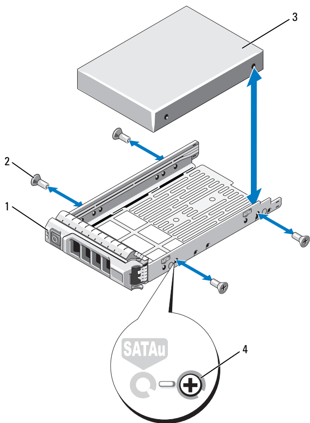
图 3-8. 将硬盘驱动器安装到驱动器托盘中
