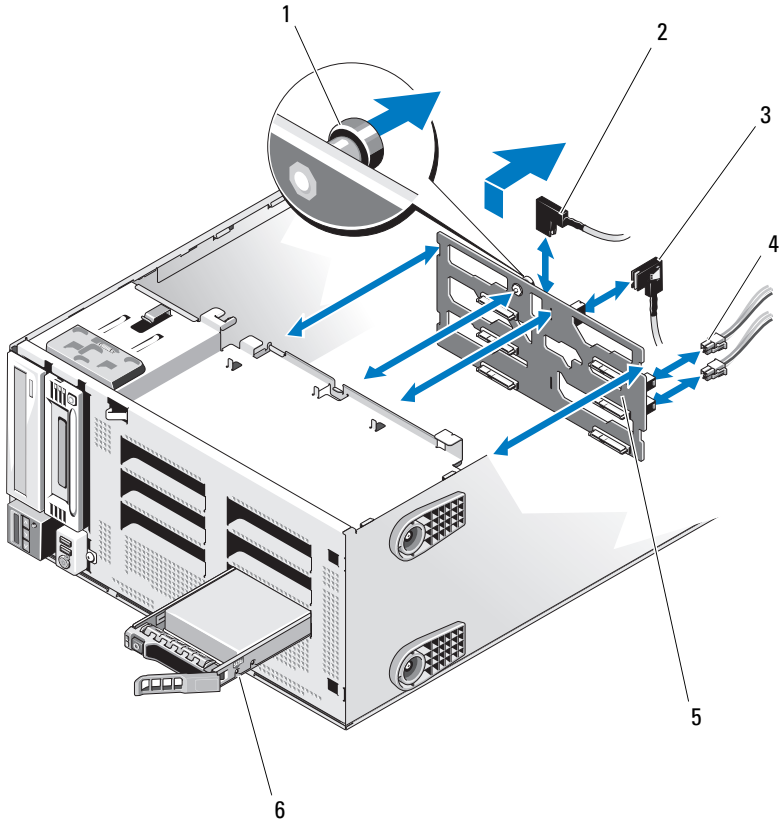
图 3-27. 卸下和安装 SAS 背板
