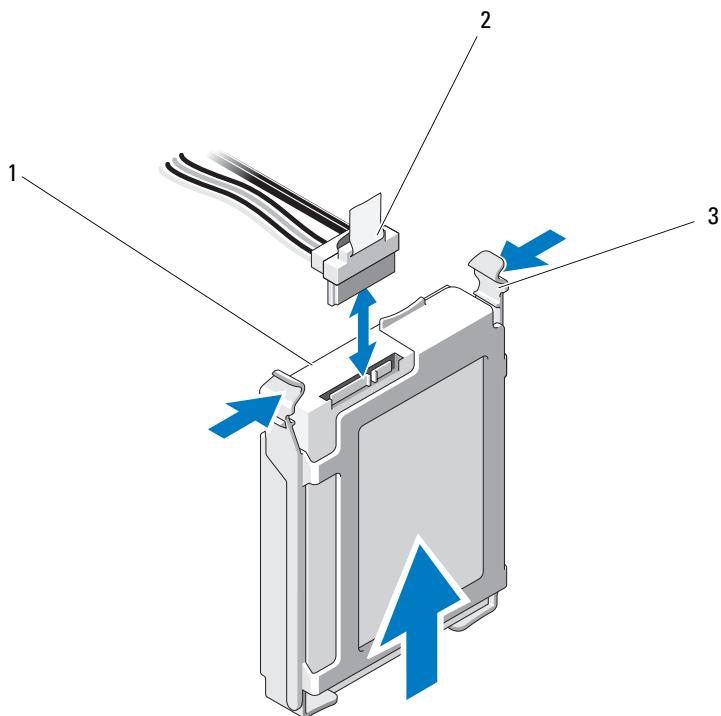
图 3-9. 卸下和安装已连接电缆的硬盘驱动器
