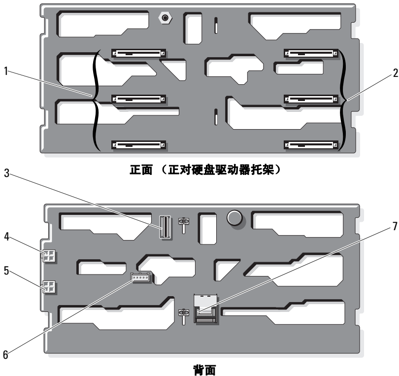
图 6-2. SAS 背板连接器
