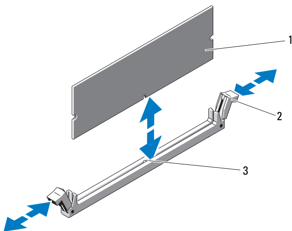
图 3-13. 安装和卸下内存模块
