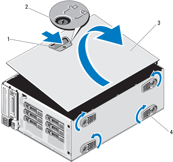
图 3-5. 打开与合上系统护盖
