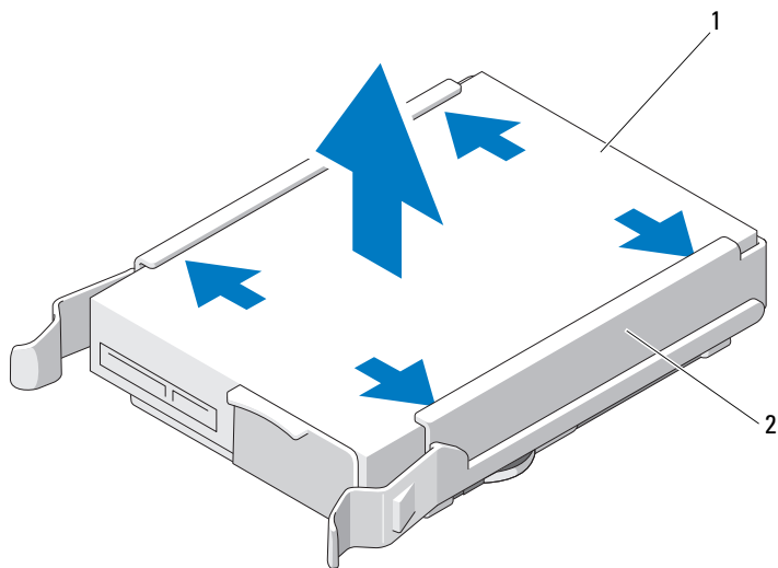
图 3-10. 从硬盘驱动器支架中卸下硬盘驱动器
