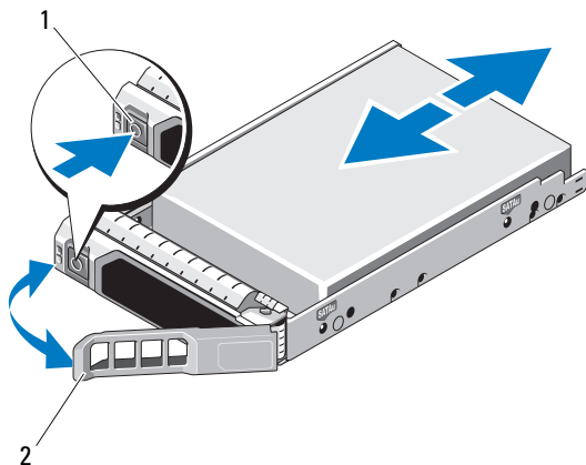
图 3-7. 卸下和安装可热插拔的硬盘驱动器
