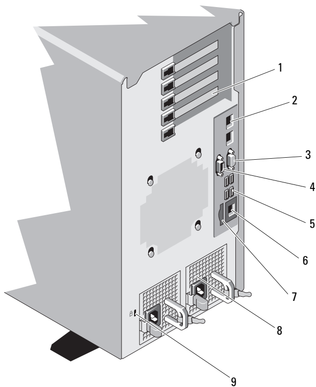
图 1-4. 背面板部件和指示灯
